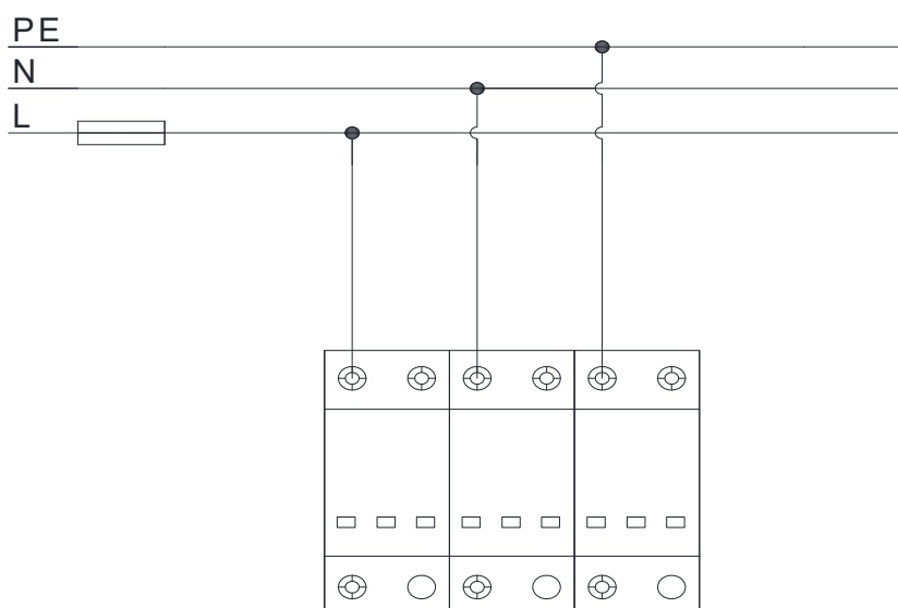
单相电源推荐2+1接法
