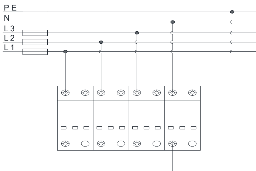
对地保护接线法
