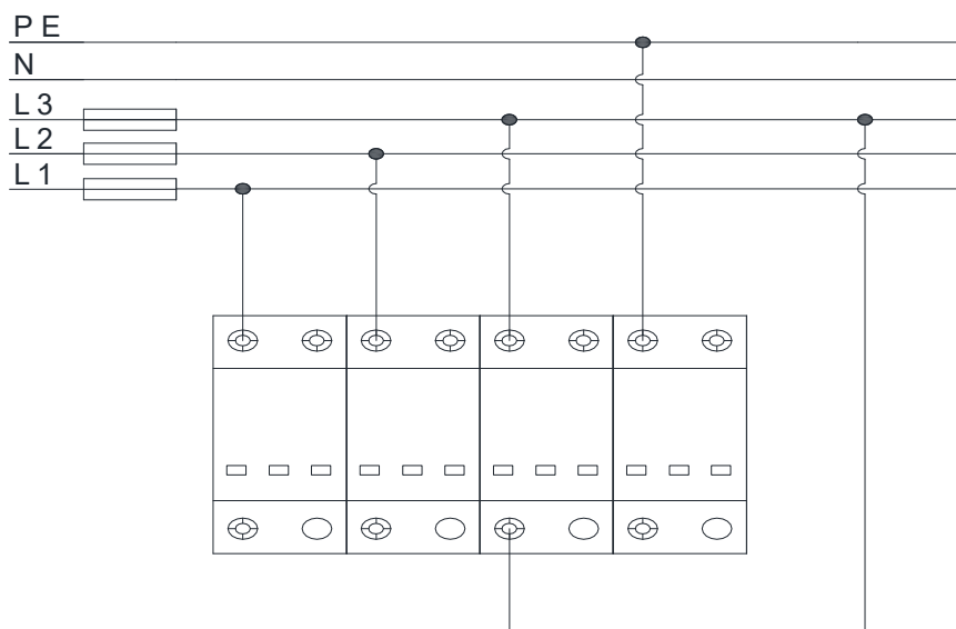
3+NPE 零地保护接线法
