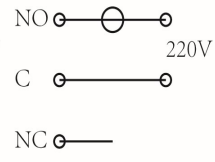
远端点亮报警灯
