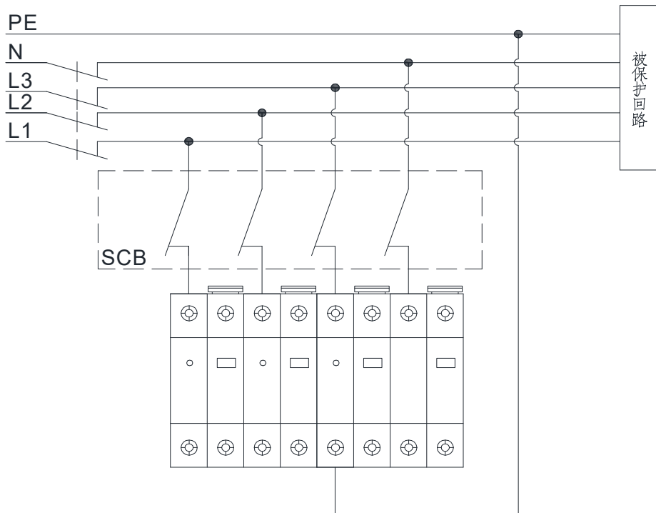
4P 接线示意图
