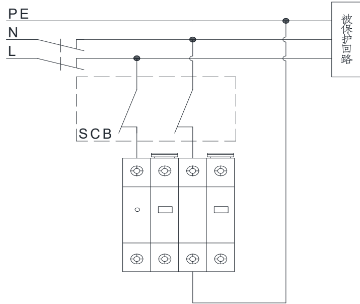
2P 接线示意图
