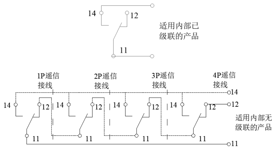
遥信输出接线方式示意图
