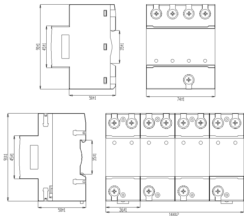
产品尺寸图
