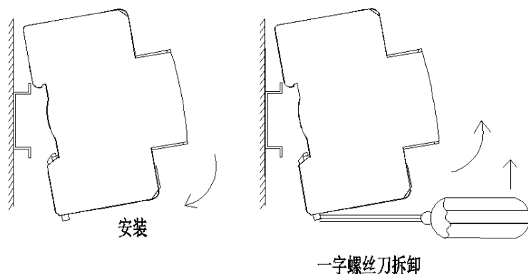
产品安装和拆卸方式图
