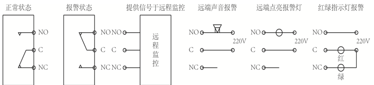
遥信输出接线方式示意图
